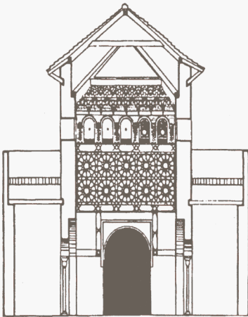
Sección del Pabellón Central. Fuente: "El Cuarto Real de Sto. Domingo de Granada". Basilio Pavón Maldonado.
