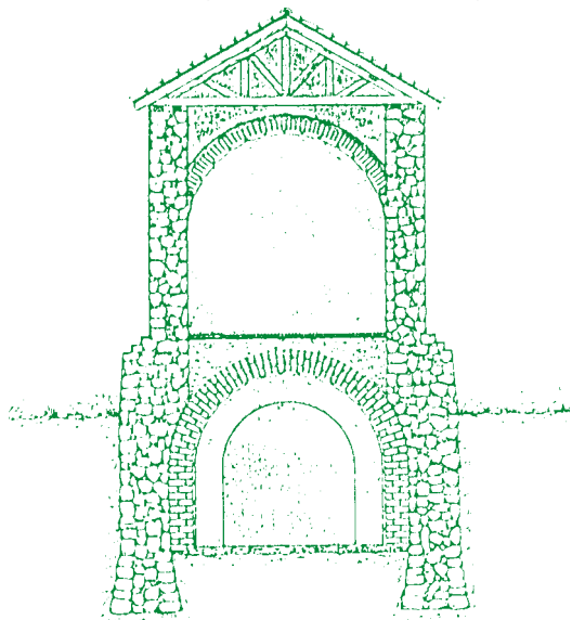
Reconstrucción ideal según R. Puertas
