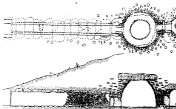
Planta y alzado de S. Giménez Reyna
