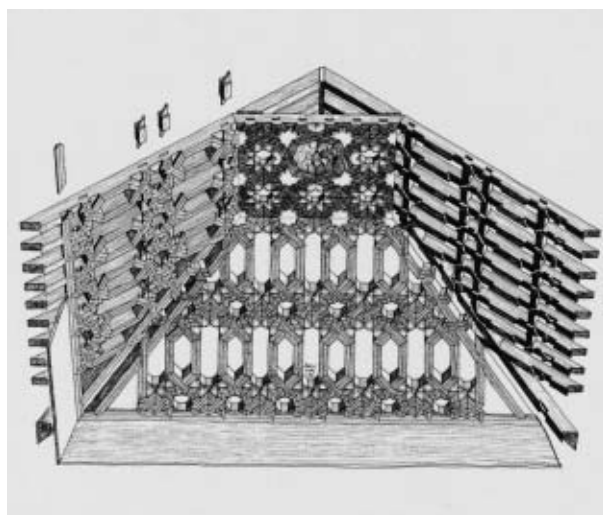
Armadura
