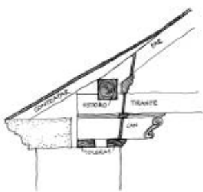
Esquema de la solera de una armadura
