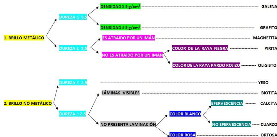
CLAVE SENCILLA DE IDENTIFICACIÓN DE MINERALES.
